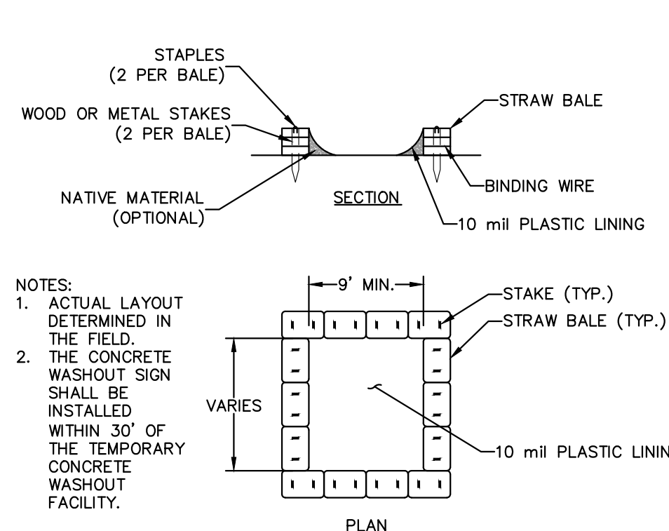
CONCRETE & STUCCO WASTE MANAGEMENT N.T.S.
