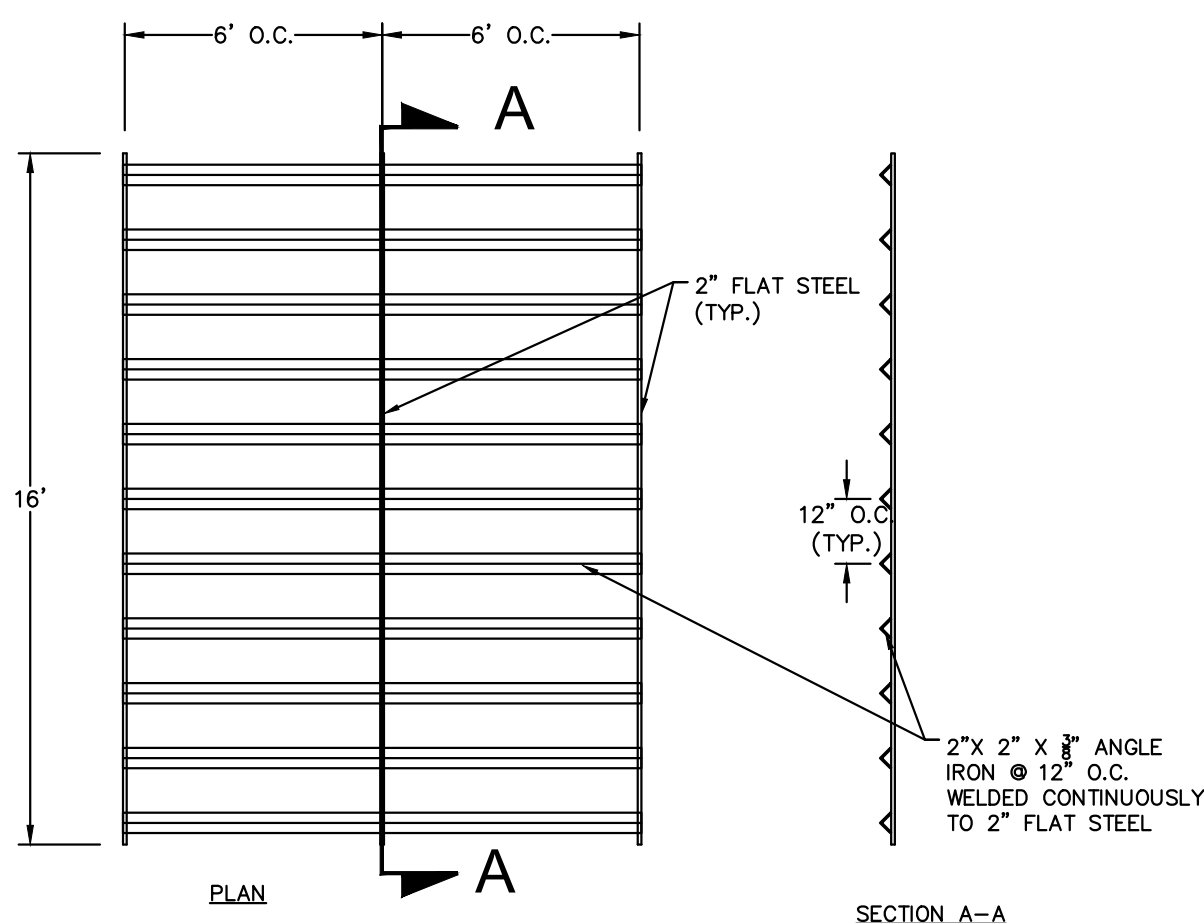
WASH RACK N.T.S.
